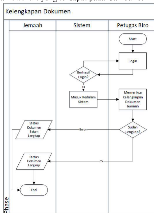
Gambar 5 Flowchart kelengkapan dokumen
